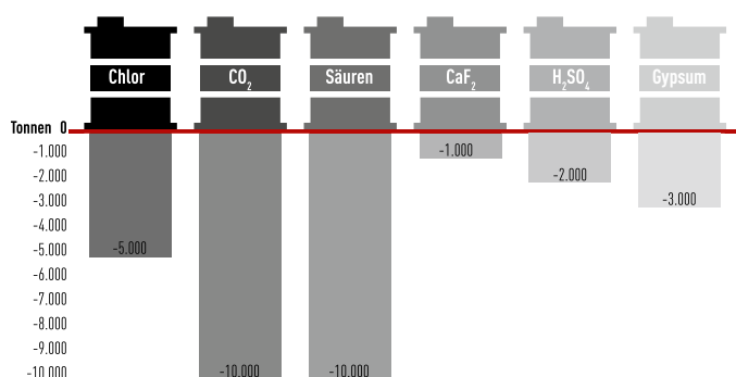
Bild 3: Die Umweltentlastung pro 1.000 Tonnen upcycliertes Monomer TFE ist enorm. Unerwünschte Nebenprodukte des regulären Monomer-Herstellungsprozesses, wie CO 2 und Salzsäure, werden dabei sogar komplett vermieden.
